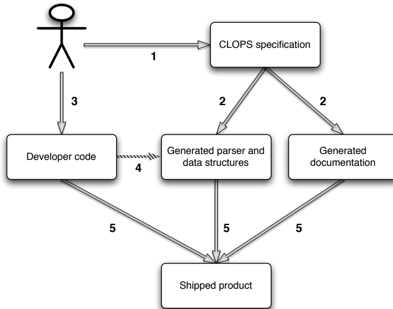
Fig. 1. Developer usage scenario.
